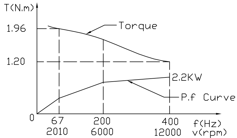
扭矩/功率曲线
